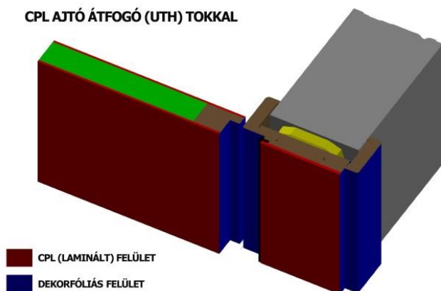
CPL AJTÓ GERÉB TOKKAL
