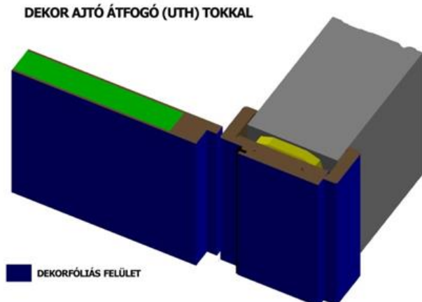
DEKOR AJTÓ ÁTFOGÓ (UTH) TOKKAL
