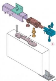
Tolóajtó vasalat szerkezeti felépítése és alkatrészei
