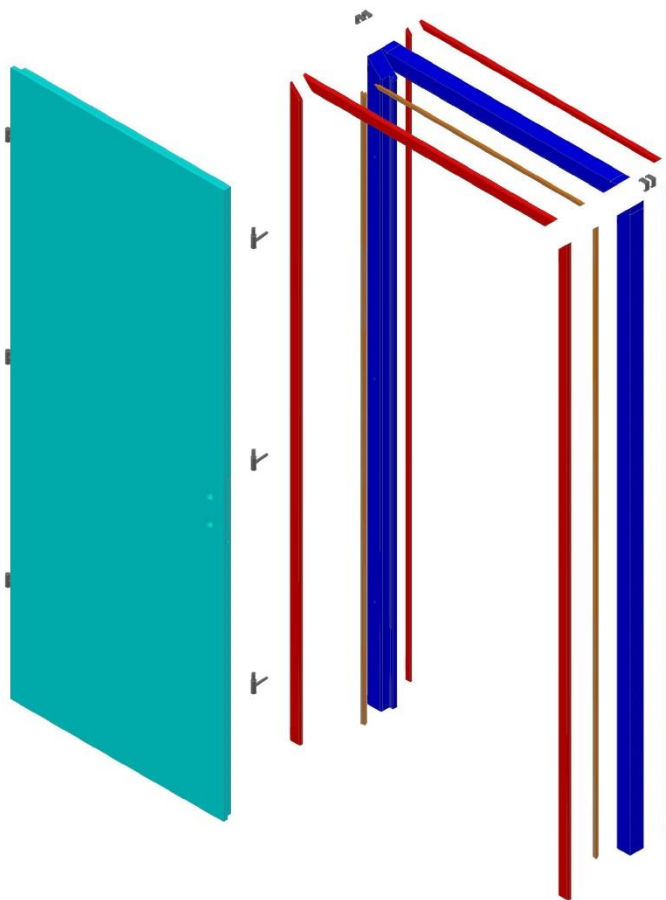
Gerébtokos ajtó robbantott rajza
